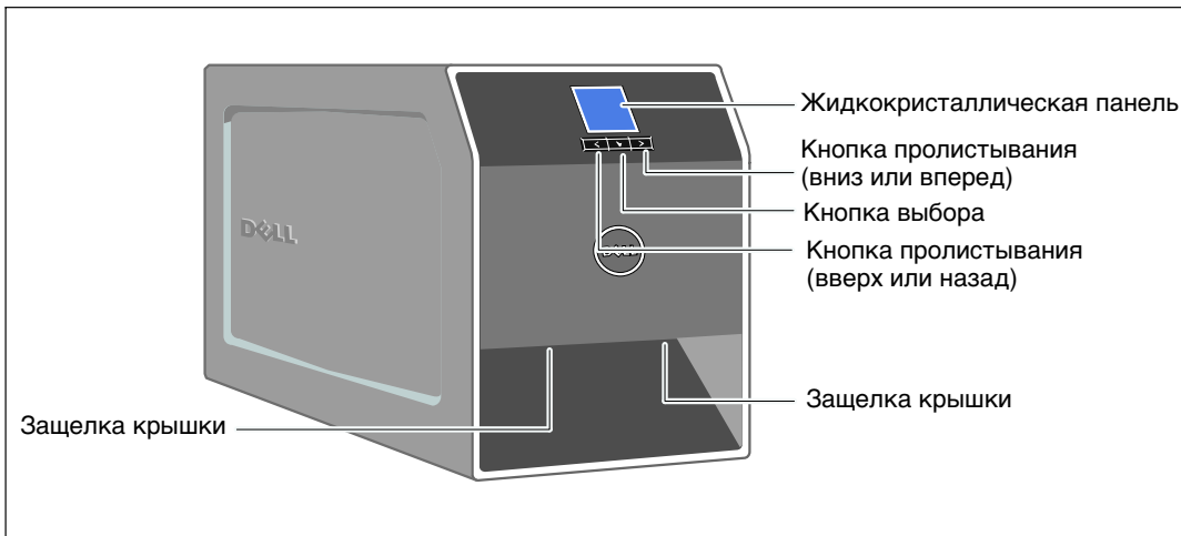
Рис. 9. ИБП "Башня" Dell
