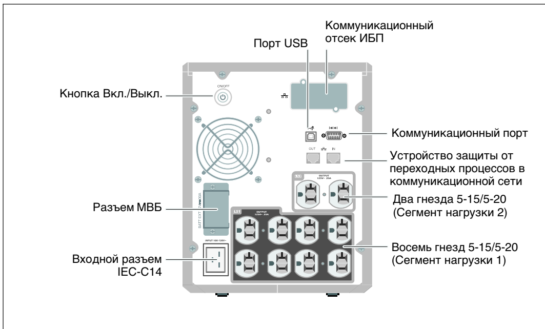
Рис. 7. Задняя панель 1920 Вт / 120В, 1500Вт / 100 В
