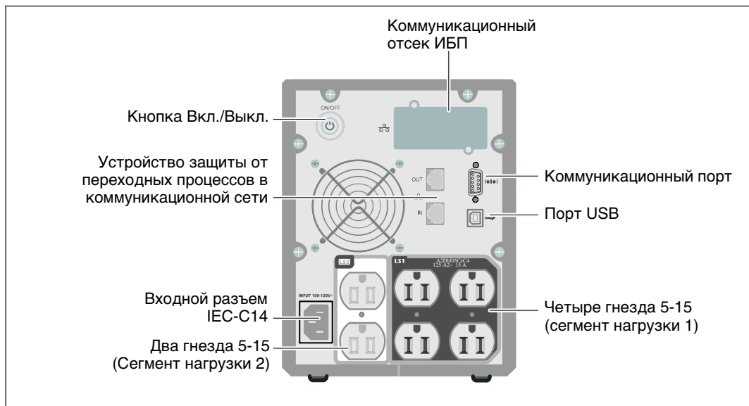
Рис. 3. Задняя панель 500 Вт, 100/120 В
