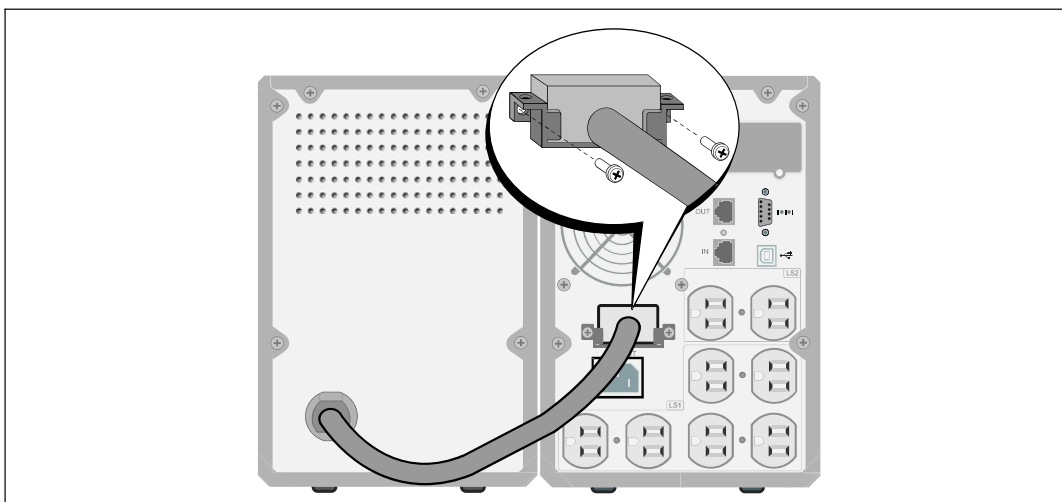
Рис. 15. МВБ Установка только для моделей ИБП "Башня" 1000 Вт и 1920/1500 Вт
