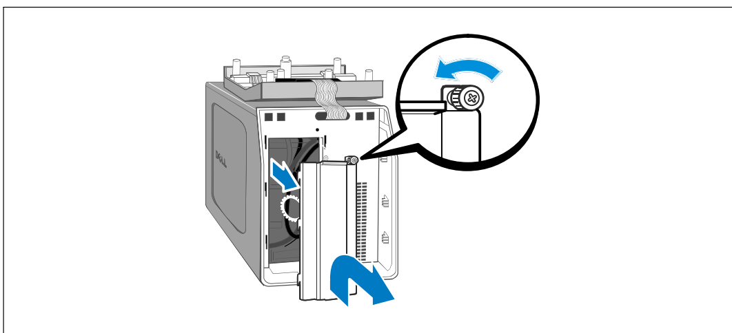
Рис. 11. Снятие крышки батарей
