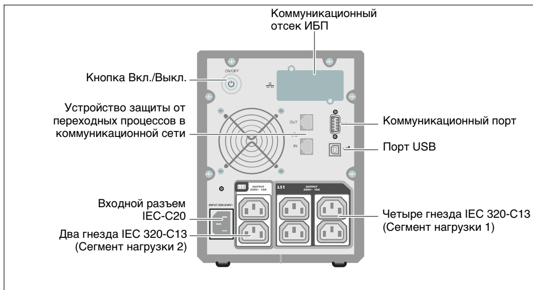
Рис. 4. Задняя панель 500 Вт, 230 В
