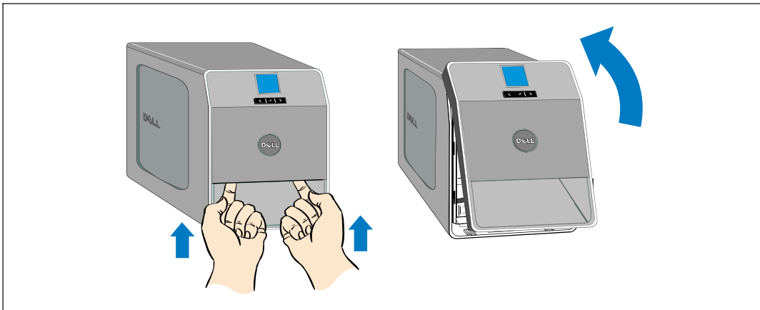
Рис. 24. Снятие передней крышки ИБП
