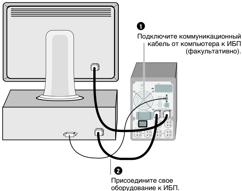
Рис. 16. Установка типичного ИБП (показана модель 120 В)
