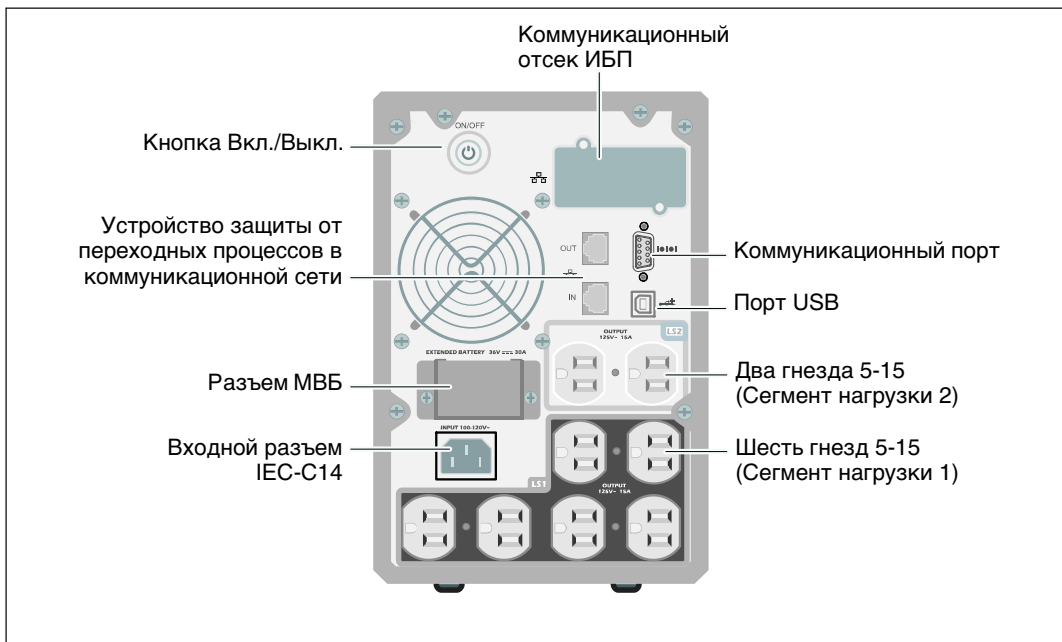
Рис. 5. Задняя панель 1000 Вт, 120 В
