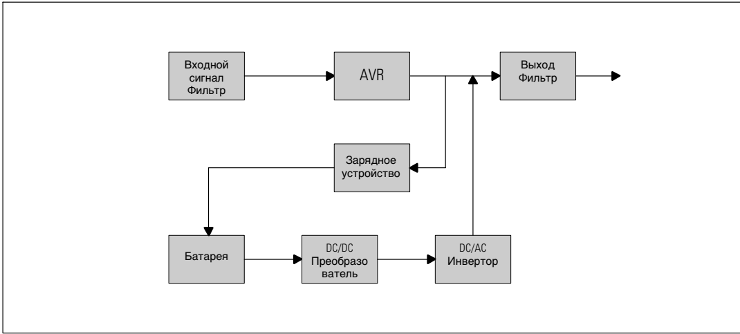
Рис. 27. Блок-схема линейно-интерактивного ИБП
