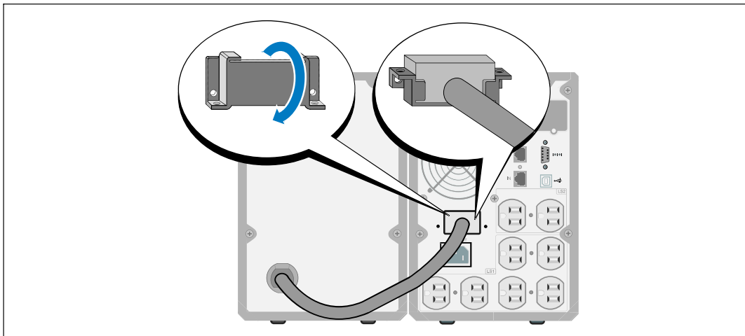
Рис. 14. Установка крышки разъема батарей
