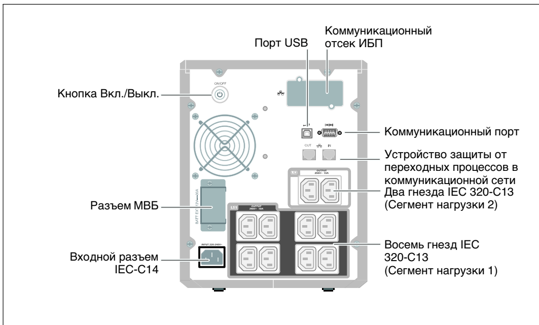
Рис. 8. Задняя панель 1920 Вт, 230 В
