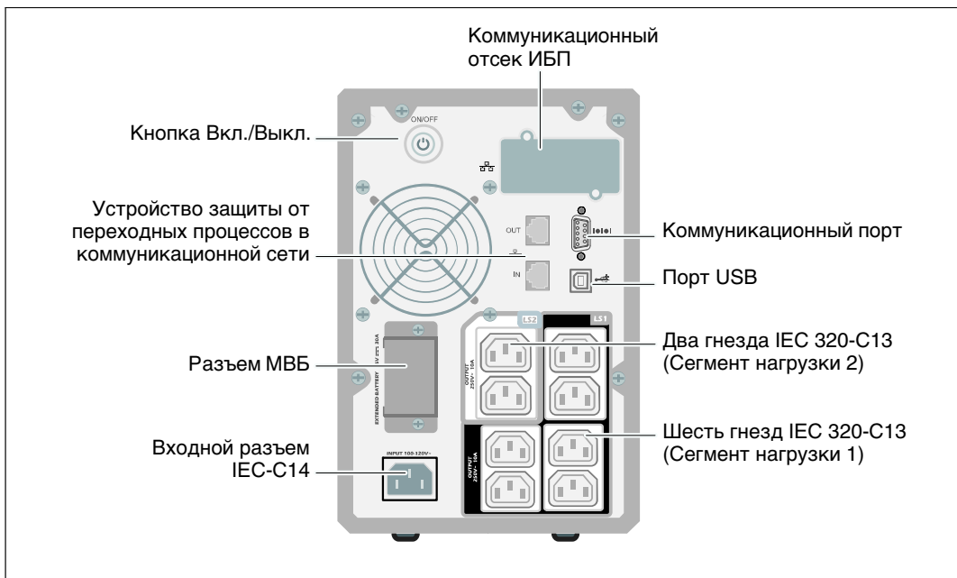
Рис. 6. Задняя панель 1000 Вт, 230 В
